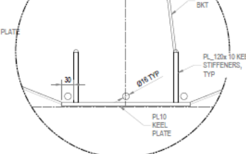
DETAIL 2 - KEEL
